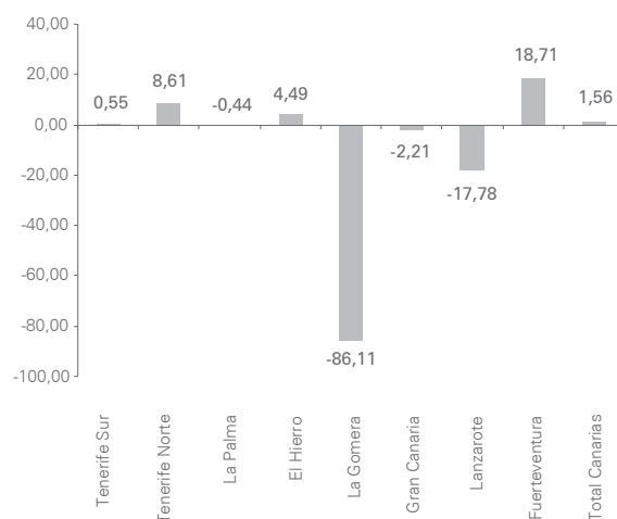
TASA DE VARIACIÓN TRÁFICO DE MERCANCÍAS POR LOS AEROPUERTO CANARIOS 2006-2007
