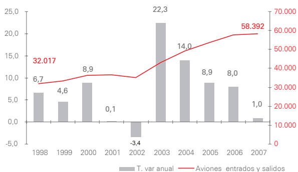
TRÁFICO COMERCIAL DE AVIONES EN EL AEROPUERTO TENERIFE NORTE 1998-2007
